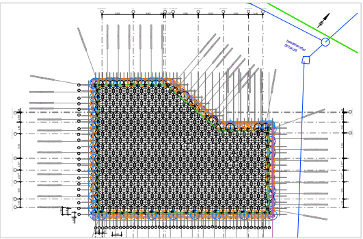
Injektionsplan von PORR Spezialtiefbau Planung GmbH
